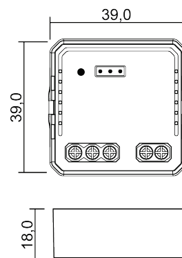
Senza clip di montaggio
