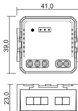
Con clip di montaggio
