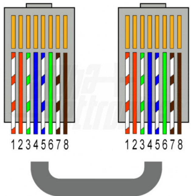
Connessione EIA568B
